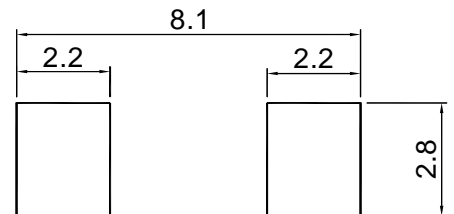
LL-41 (MELF) DO-213AB (MELF)
