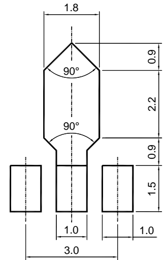
SOT-89
