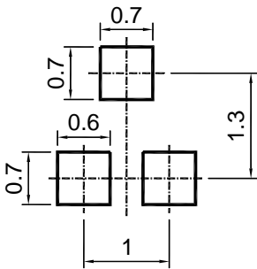
SOT-523
