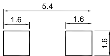
LL-34 (Mini MELF) DO-213AA (Mini MELF) LS-34 (Quadro MELF)
